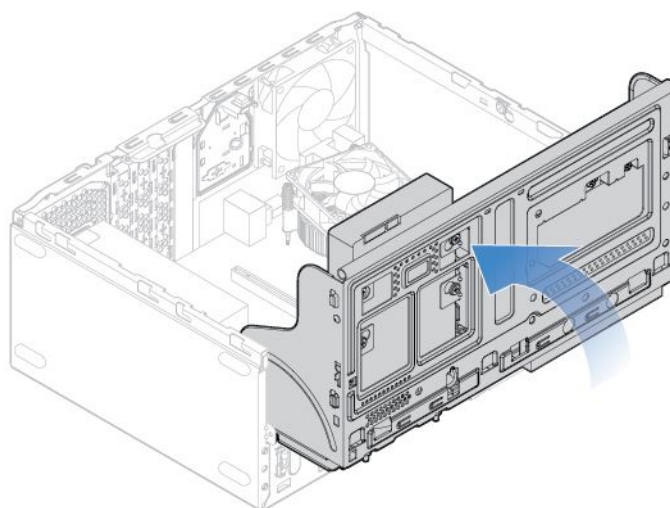
图 75. 向下旋转驱动器托架组合件
