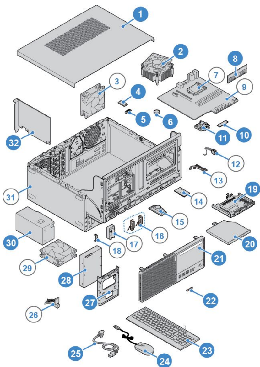
图 7. 确定 FRU 的位置 (包括 CRU)
