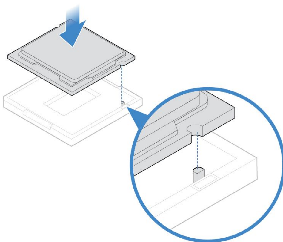
图 83. 安装微处理器
