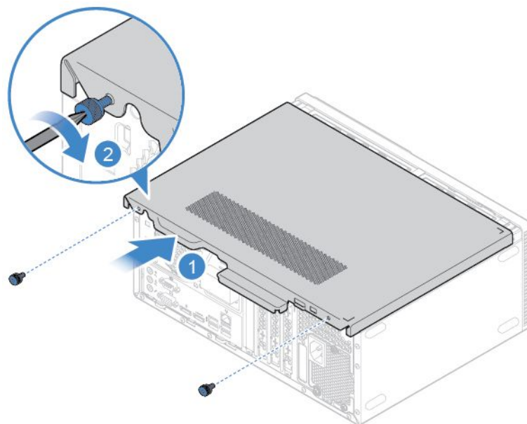
图 88. 重新安装计算机外盖
