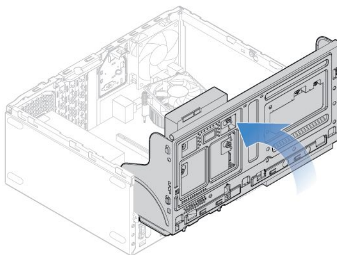
图 16. 向下旋转驱动器托架组合件
