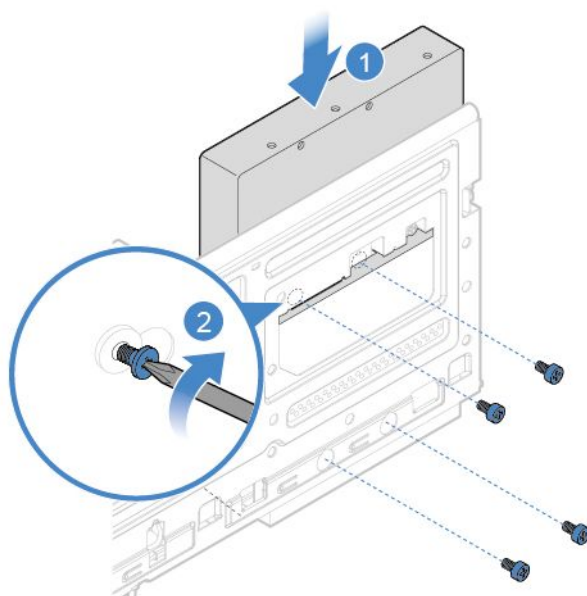
图 20. 安装 3.5 英寸辅助存储驱动器
