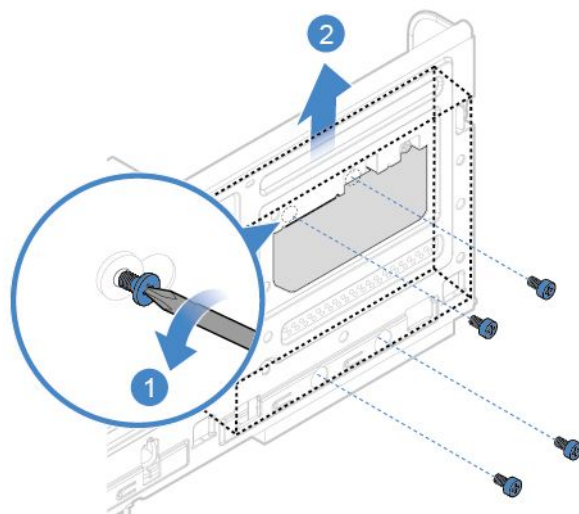
图 19. 卸下 3.5 英寸辅助存储驱动器
