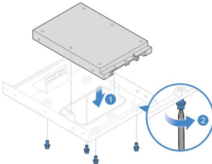
图 22. 将 2.5 英寸存储驱动器装入存储转换装置
