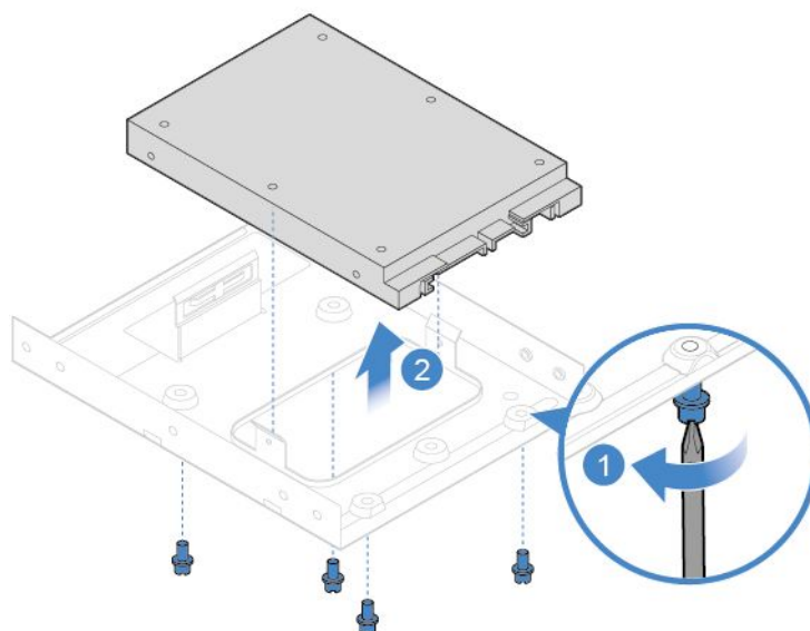
图 21. 从存储转换装置上卸下 2.5 英寸存储驱动器
